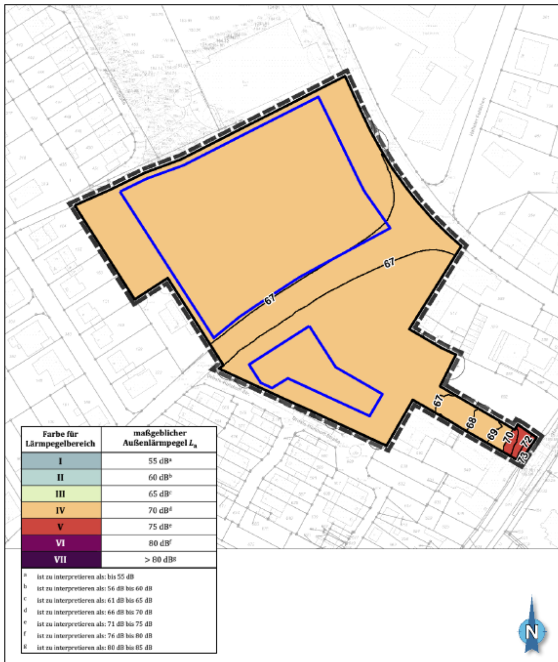
Abbildung 7.8: Lärmpegelbereiche/Außenlärmpegel nach DIN 4109, M = 1 : 1.900, schutzbedürftige Räume (mit oder ohne Schlafnutzung)
